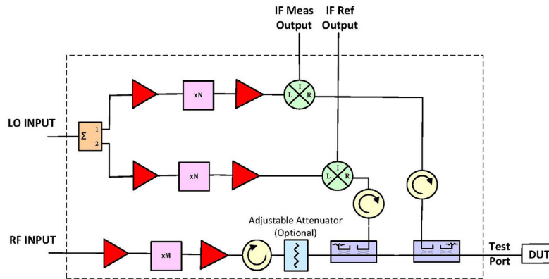
Fig. 2 - TX/RX Extender
