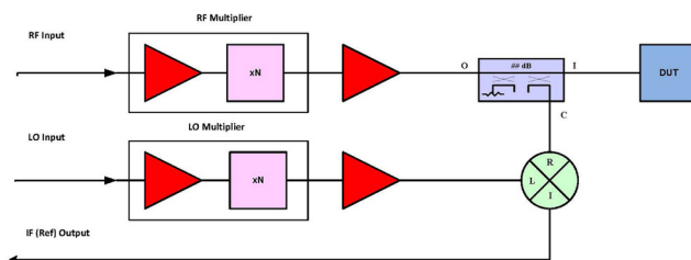
Fig. 4 - TX/REF Extender
