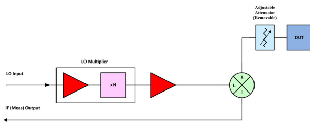
Fig. 3 - RX Extender
